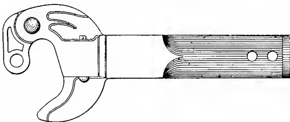
Fig. 2151. Plan.
